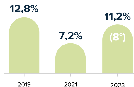
Gráfico 9. Desocupación, 2019 - 2023
