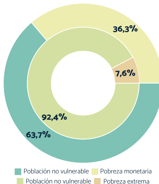
Gráfico 2. Pobreza monetaria, 2023
